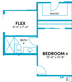
Optional Bedroom 4 and Bath 4 in lieu of Tandem Garage
