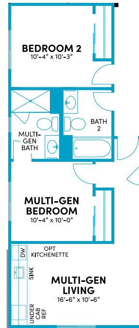
Optional Multi-Gen Suite
