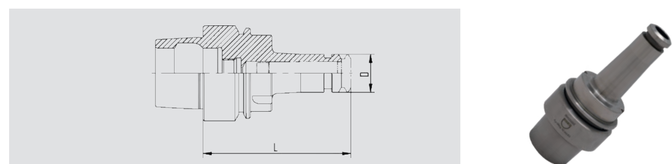
HSK 40 HSK Werkzeugaufnahme mit Kern Spezialdesign ähnlich HSK-E40
