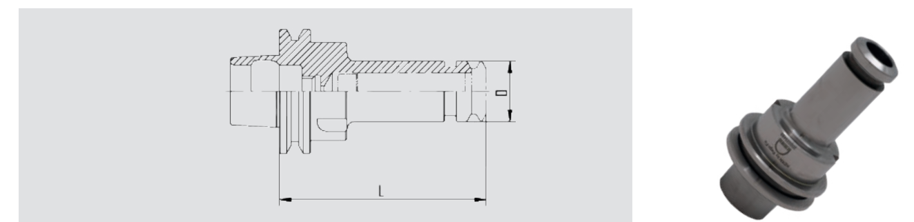
HSK 25 HSK Werkzeugaufnahme mit Kern Spezialdesign ähnlich HSK-E25
