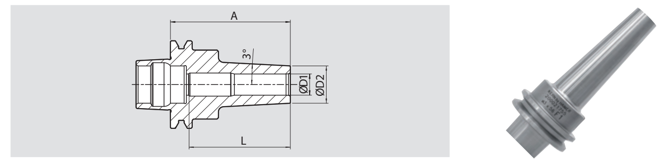
HSK 25 Mini-Shrink HSK Werkzeugaufnahme mit Kern Spezialdesign ähnlich HSK-E25
