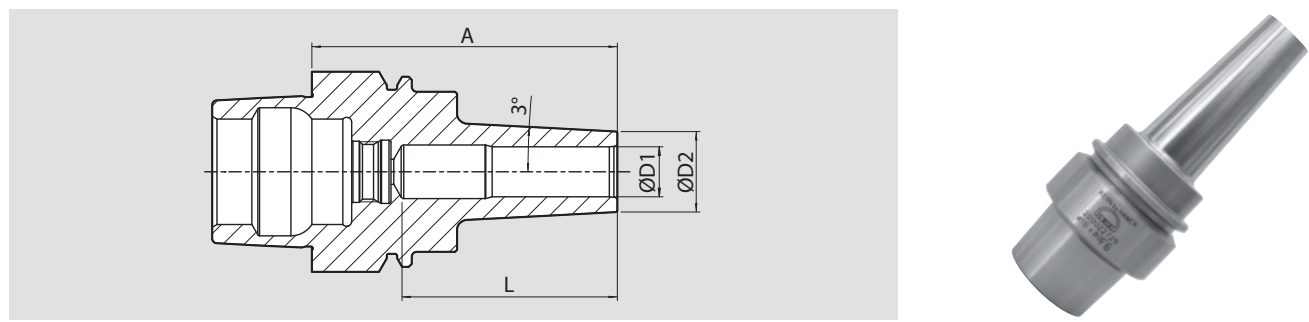
HSK 40 Mini-Shrink HSK Werkzeugaufnahme mit Kern Spezialdesign ähnlich HSK-E40
