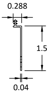
103) NAIL FIN VINYL
