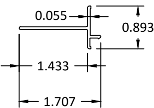
70) NAIL FIN ALUMINUM
