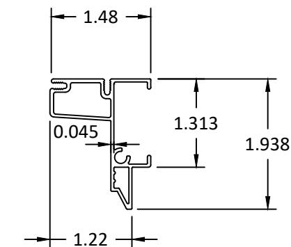
57) STD. FRAME CLADDING
