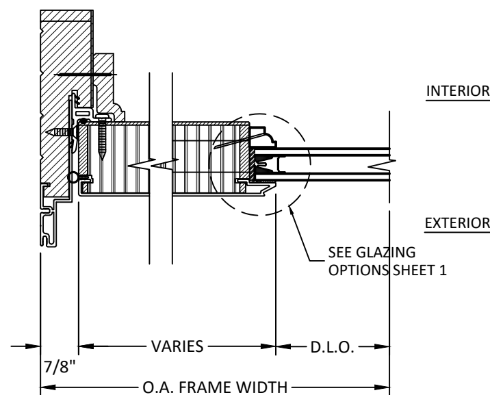
4 4.0 HORIZONTAL SECTION SIDELITE JAMB
