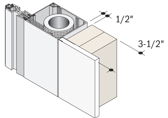
FLUSH DRYWALL
