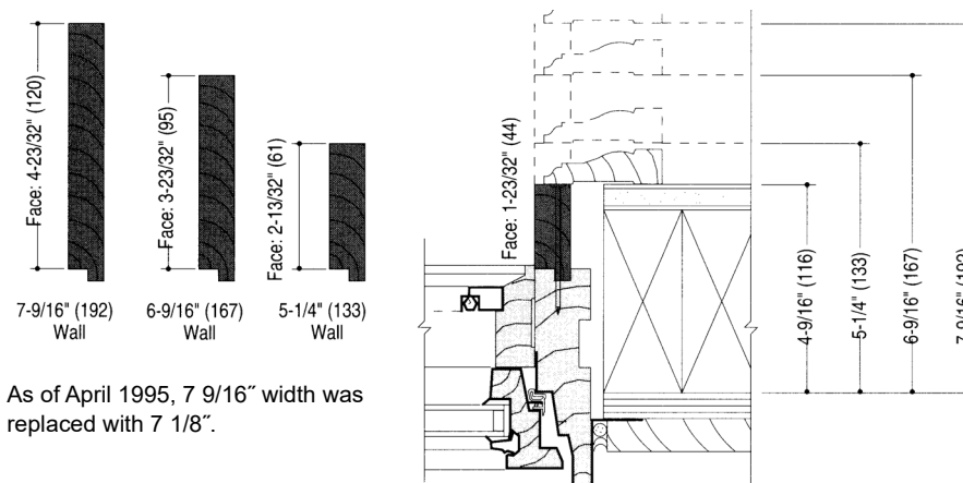
Perma-Shield® Casement Extension Jamb
