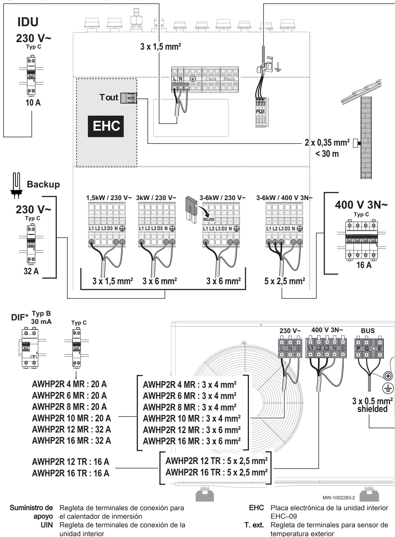
Fig.69 Esquema de cableado y secciones transversales de cable recomendadas
