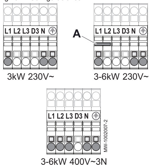
Fig.79 Configuraciones
