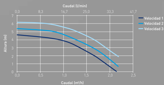
Platinum BC Monobloc 10
