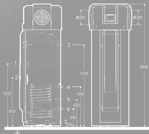
BC ACS 300 1 E (mm)
