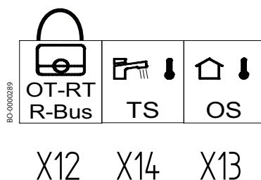
Fig.28 Conexión del termostato de ambiente (OT) o (R-Bus)
