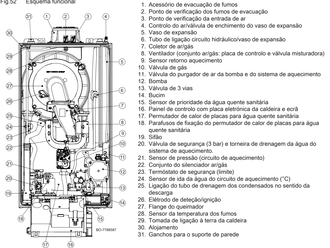
Fig.52 Esquema funcional
