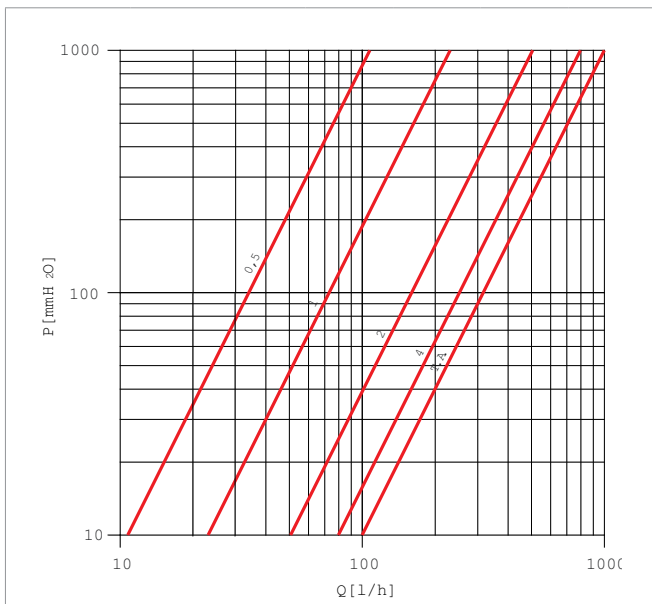
Detentor a escuadra con acabado cromado.
