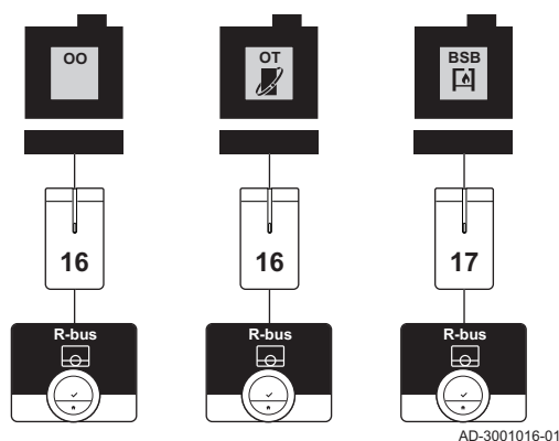
Fig.70 Pasarela con protocolos coincidentes
