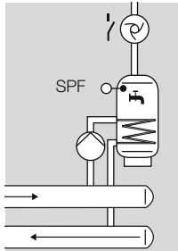
Bomba de circulación, parámetro 80 = 02
