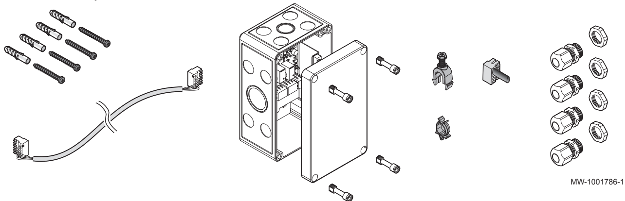
Rys.57 Zakres dostawy
