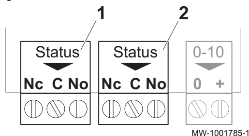
Fig.28 Relés
