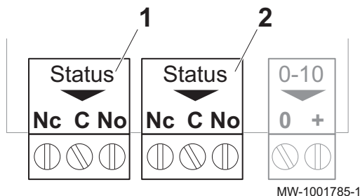
Fig.36 Relè
