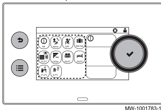
Obr.69 Ovládací panel A
