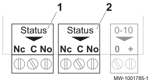
Fig.20 Relés
