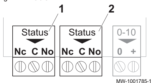
Fig.4 Relais
