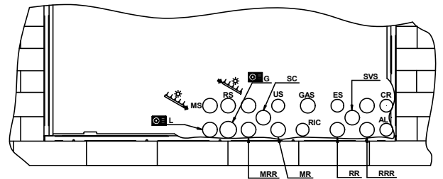
INSTALLAZIONE POSTERIORE (vista frontale)
