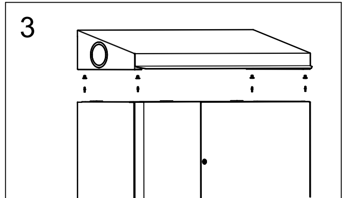
Agganciare la copertura sopra l'armadio facendo attenzione ad allineare le clips con i piolini.
