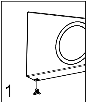
Inserire le 4 clips di fissaggio copertura nelle apposite asole;
