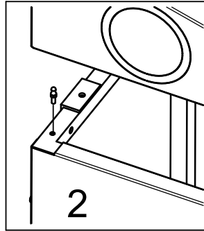
Avvitare i piolini negli appositi fori filettati predisposti nel telaio dell'armadio;
