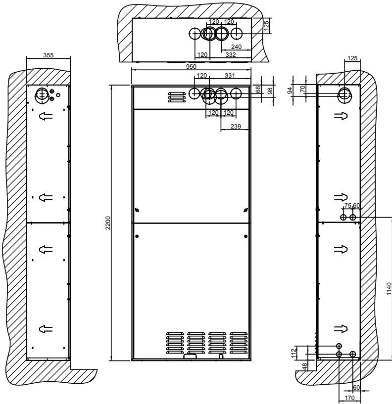
Cassa di contenimento Acqua Più 150 (versione 300)
