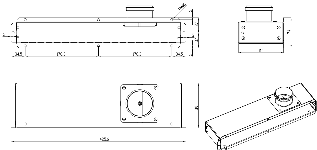
A7767627 PL MET RB 1xDN75
