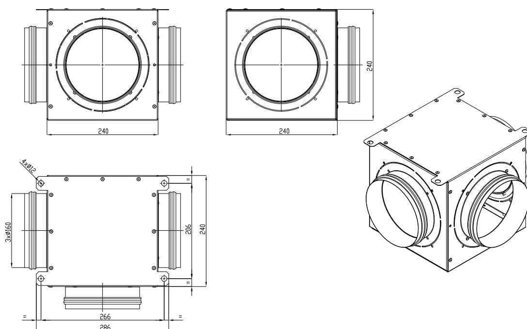
A7767610 PL DIS. 3T 3x160mm
