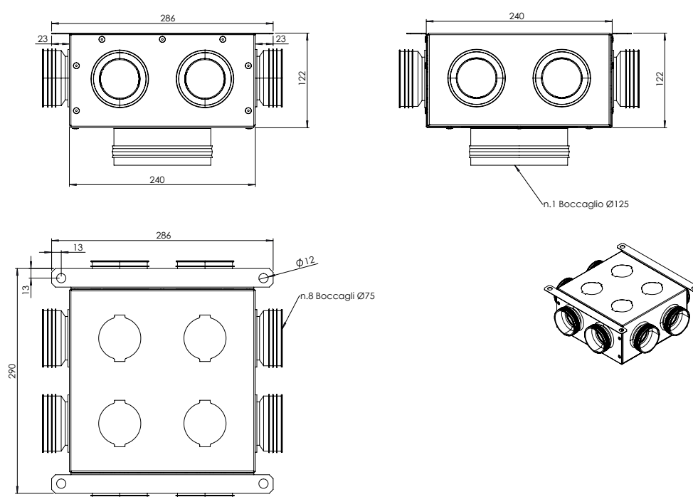
A7841461 PL. DIS. BX 8xDN90 D.125mm
