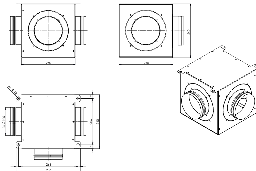
A7841466 PL. DIS. 3T 3x125mm
