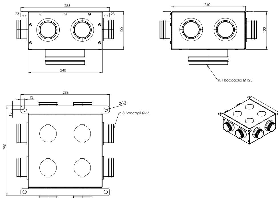
A7841460 PL. DIS. BX 8xDN75 D.125mm
