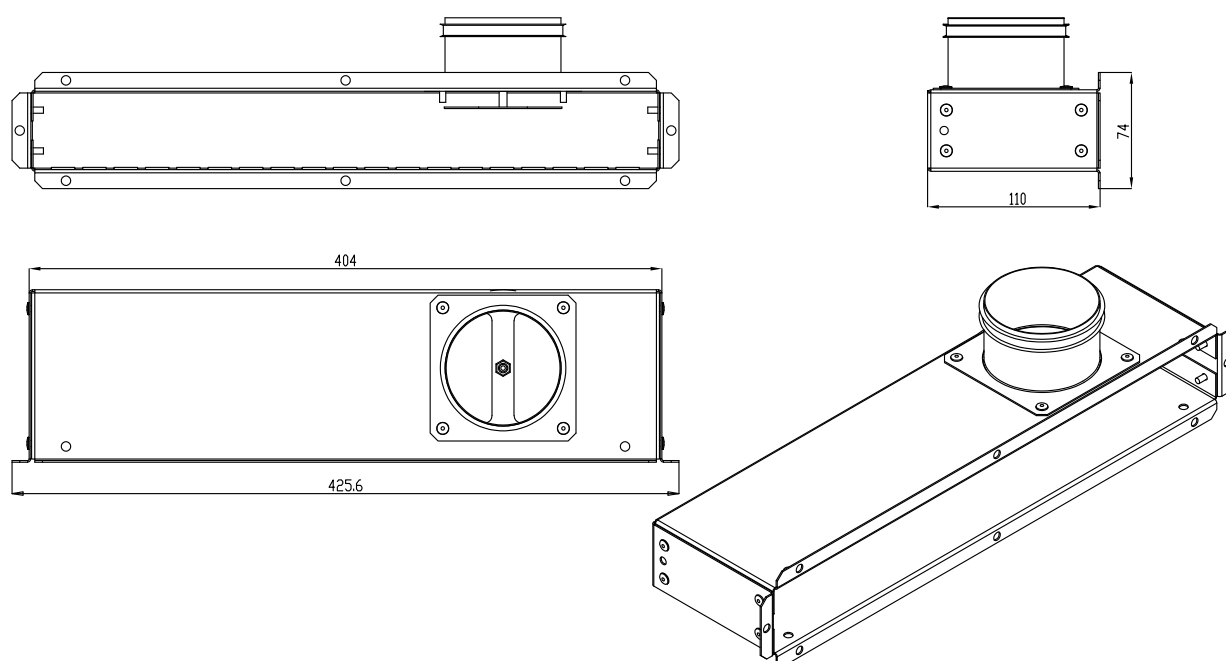
A7767628 PL MET RB 1xDN90
