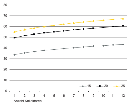
Druckverlust C 250 Kollektoren
