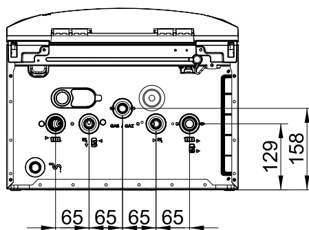
Onderaanzicht
