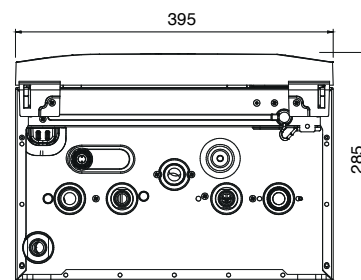
Onderaanzicht
