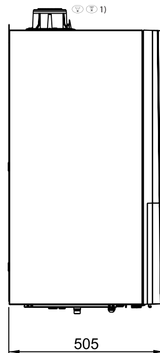
Rechterzij aanzicht
