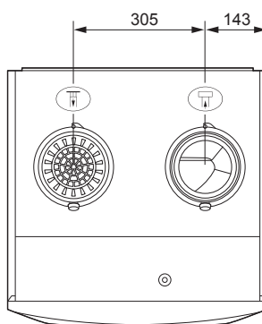
Bovenaanzicht
