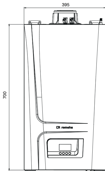
Vooraanzicht
