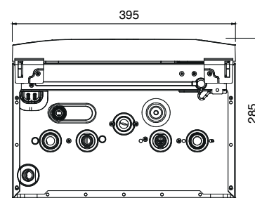
Onderaanzicht
