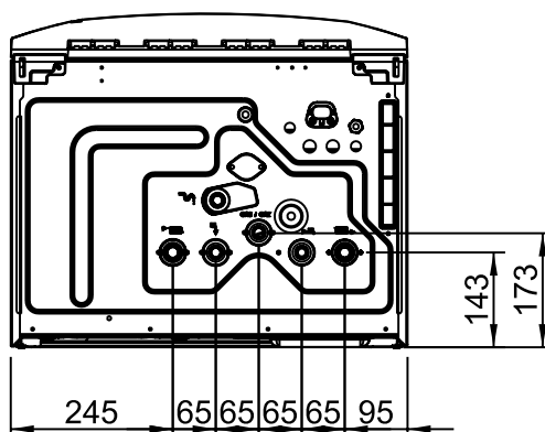
Onderaanzicht
