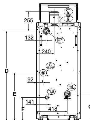
Achter aanzicht
