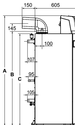
Linkerzij aanzicht
