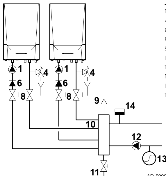
Opstellingstekening met DUO verdeler
