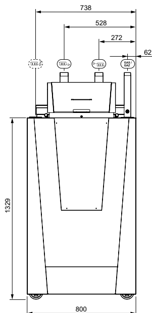
Vooraanzicht
