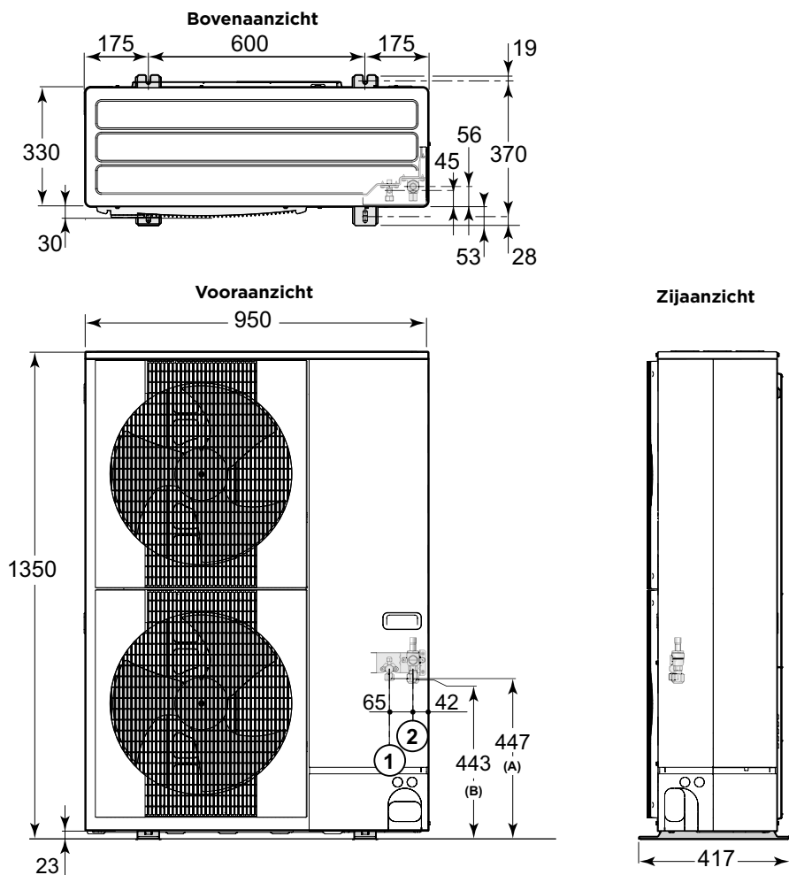
Buitendeel warmtepomp AWP 11 TR-2 | AWP 16 TR-2
