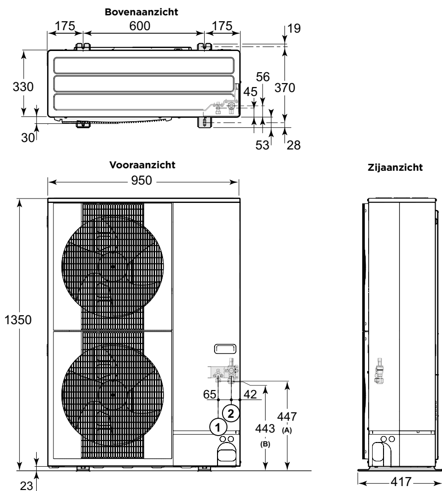
Buitendeel warmtepomp AWP R410a 11 TR-2 | AWP R410a 16 TR-2
