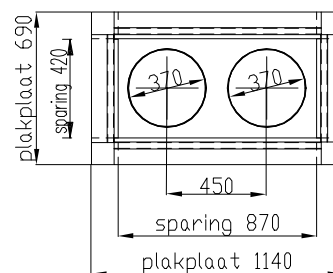
Plakplaat en sparing voor dakdoorvoer Remeha GAS 620 Ace
