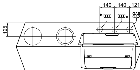
Vooraanzicht
