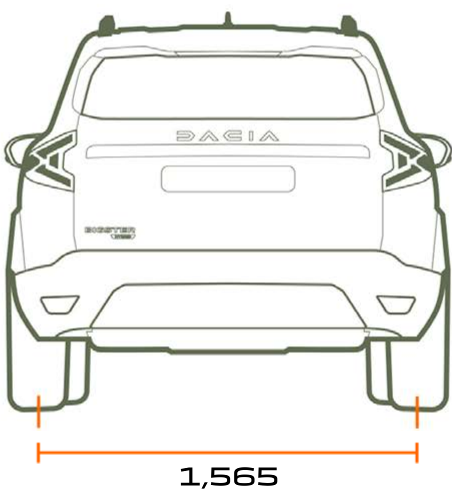
BAKIFRÅN
