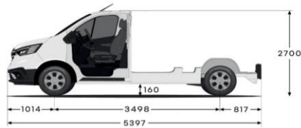
Chassi-platta
