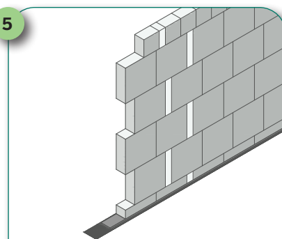
Længdekompensation
