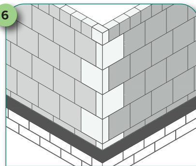
Fortanding, L-samling
