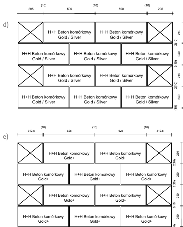
Rysunek 14. Przykładowe rozwiązanie ściany konstrukcyjnej lub działowej w zależności od materiału i szerokości ściany:
