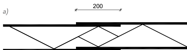
Rysunek 19. Wykonanie połączenia elementów zbrojenia typu Murfor: a) Murfor RND/Z oraz EFS/Z - minimalna długość zakładu 200 mm (zalecana 250 mm), b) Murfor Compact - minimalna długość zakładu 500 mm.
