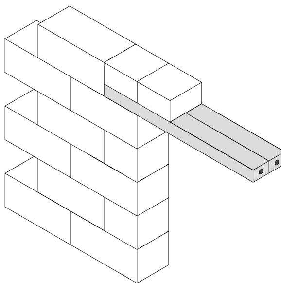
Rysunek 51. Nadproże zespolone z użyciem prefabrykatów żelbetowych.
