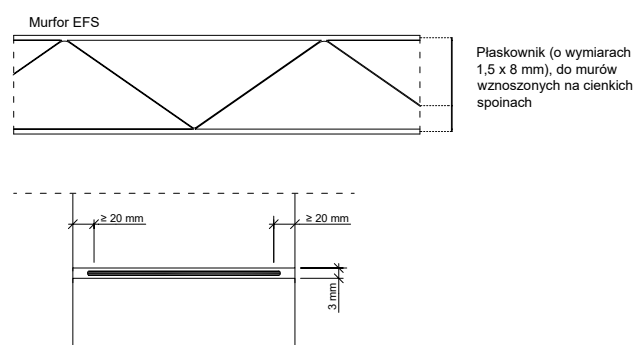
Rysunek 18. Prawidłowe ułożenie zbrojenia typu Murfor EFS/Z w spoinie wspornej cienkowarstwowej.
