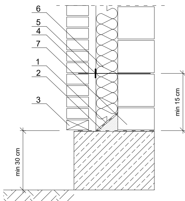
Rysunek 37. Fragment ściany szcelinowej:
