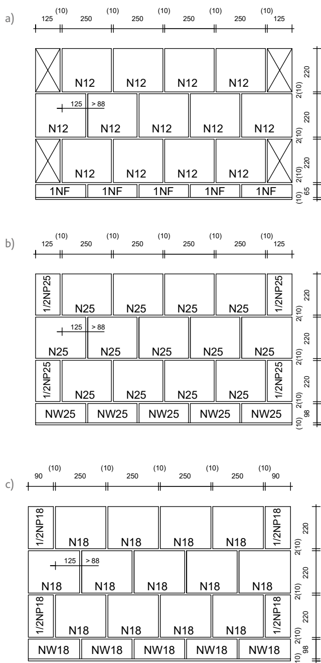
Rysunek 14. Przykładowe rozwiązanie ściany konstrukcyjnej lub działowej w zależności od materiału i szerokości ściany:
