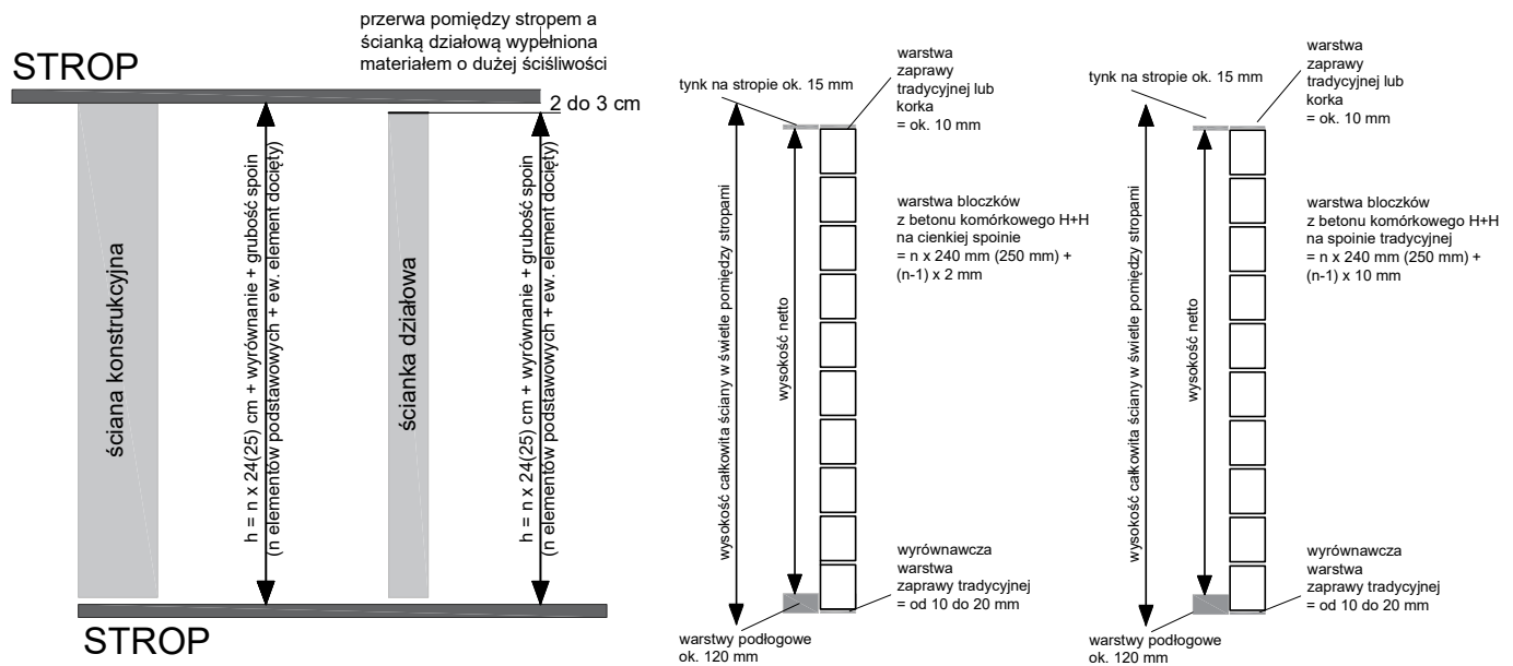
Rysunek 13. Przykładowe rozplanowanie wysokości ścian konstrukcyjnych i działowych wykonanych z H+H Betonu Komórkowego.
