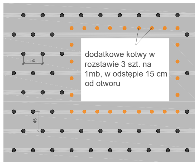
Rysunek 38. Rozmieszczenie kotew w ścianie szcelinowej.
