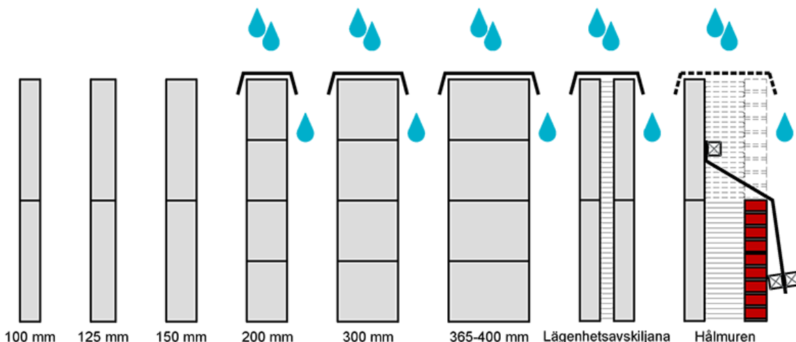
Figur 1. Skydd av murkrön, när vädret är ogynnsamt.
