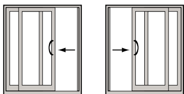
OX-Coulisse à gauche
