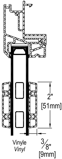
Faux-meneau avec intercalaire False mullion with spacer-bar
