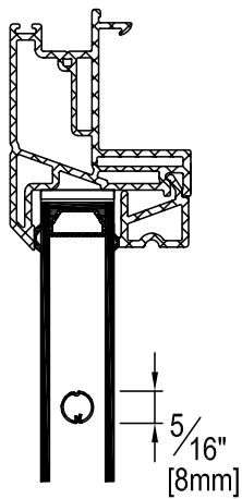
Tubulaire Pencil bar
