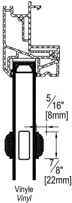
Simili barrotin avec intercalaire Simulated divided lite with spacer-bar
