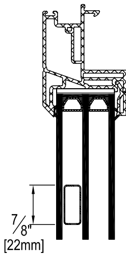
Intercalaire Spacer bar
