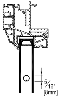
Tubulaire Pencil bar
