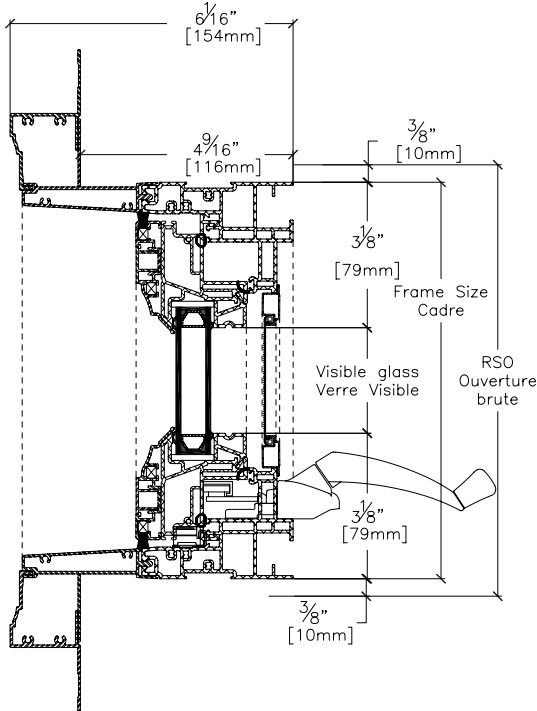
4 9/16" moulure 1 1/2" avec lame 4 9/16" 1 1/2" brickmould with flange
