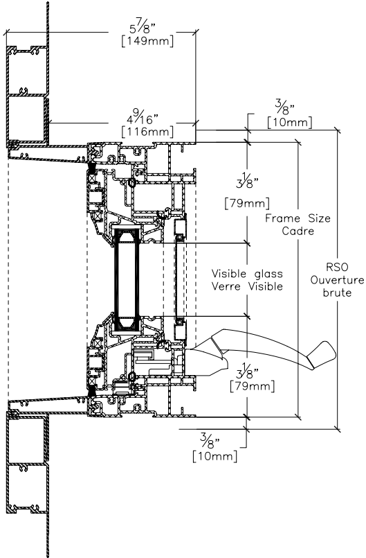
4 9/16" moulure 3 1/2" avec lame 4 9/16" 3 1/2" brickmould with flange
