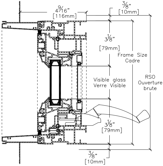
4 9/16" flush avec lame 4 9/16" flush frame with flange
