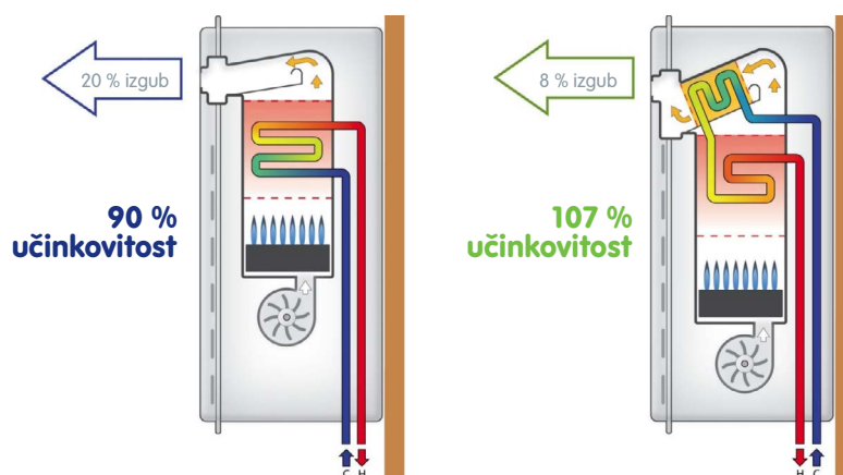
Primerjava klasičnega ter kondenzacijskega plinskega kotla.
